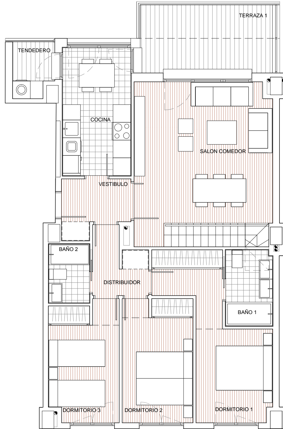
PLANTA QUINTA
