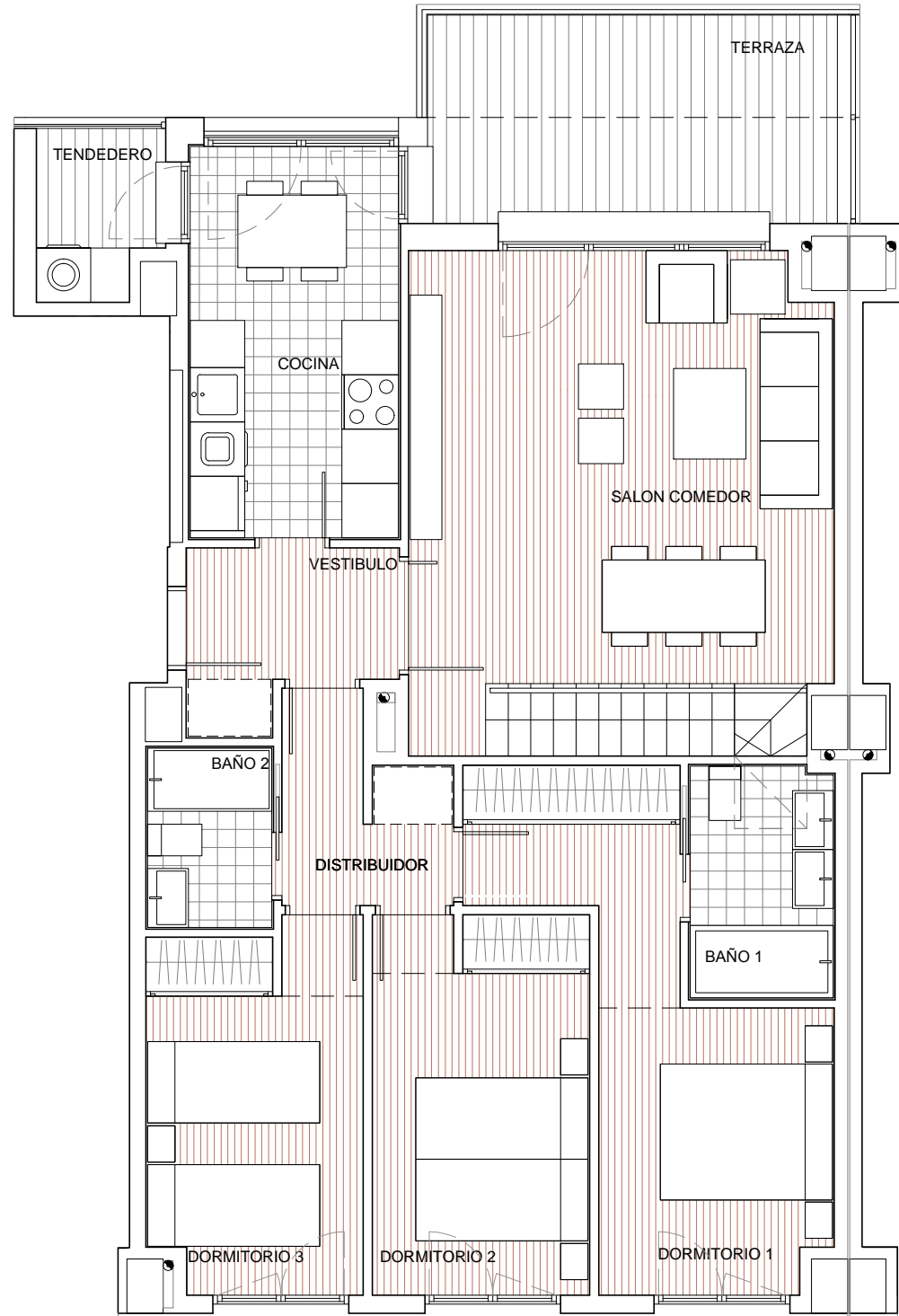
PLANTA SÉXTA
